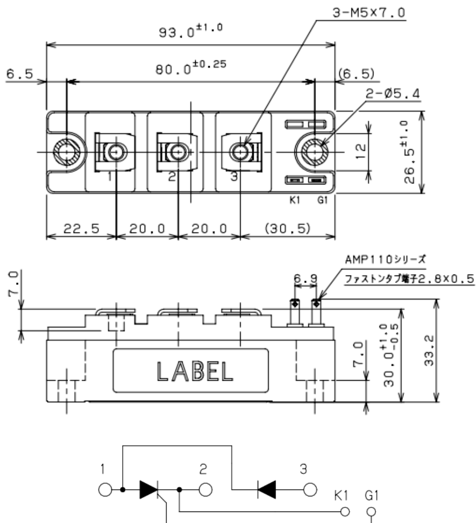
回路構成 Circuit Schema
