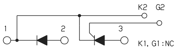
回路構成 Circuit Schema
