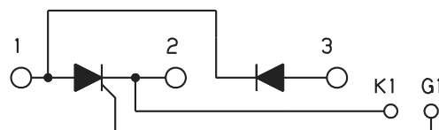
回路構成 Circuit Schema
