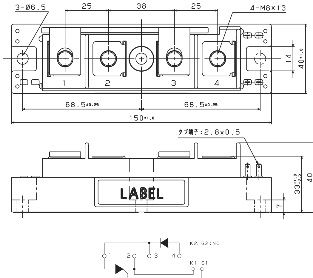
回路構成 Circuit Schema
