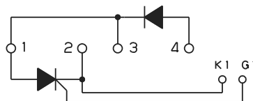
回路構成 Circuit Schema
