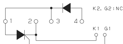
回路構成 Circuit Schema
