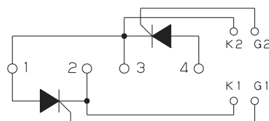
回路構成 Circuit Schema
