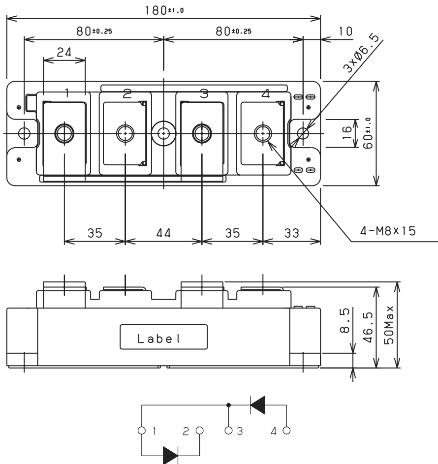
回路構成 Circuit Schema
