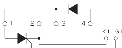
回路構成 Circuit Schema
