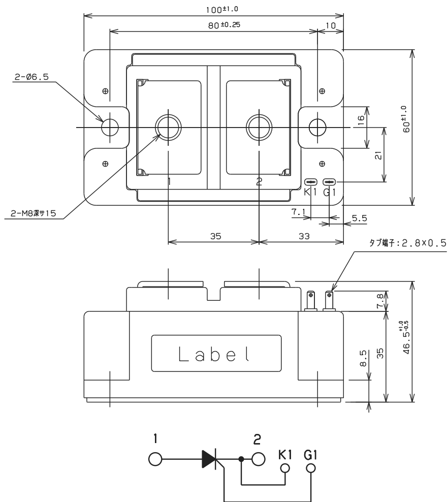
回路構成 Circuit Schema
