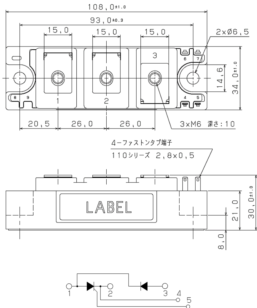
回路構成 Circuit Schema
